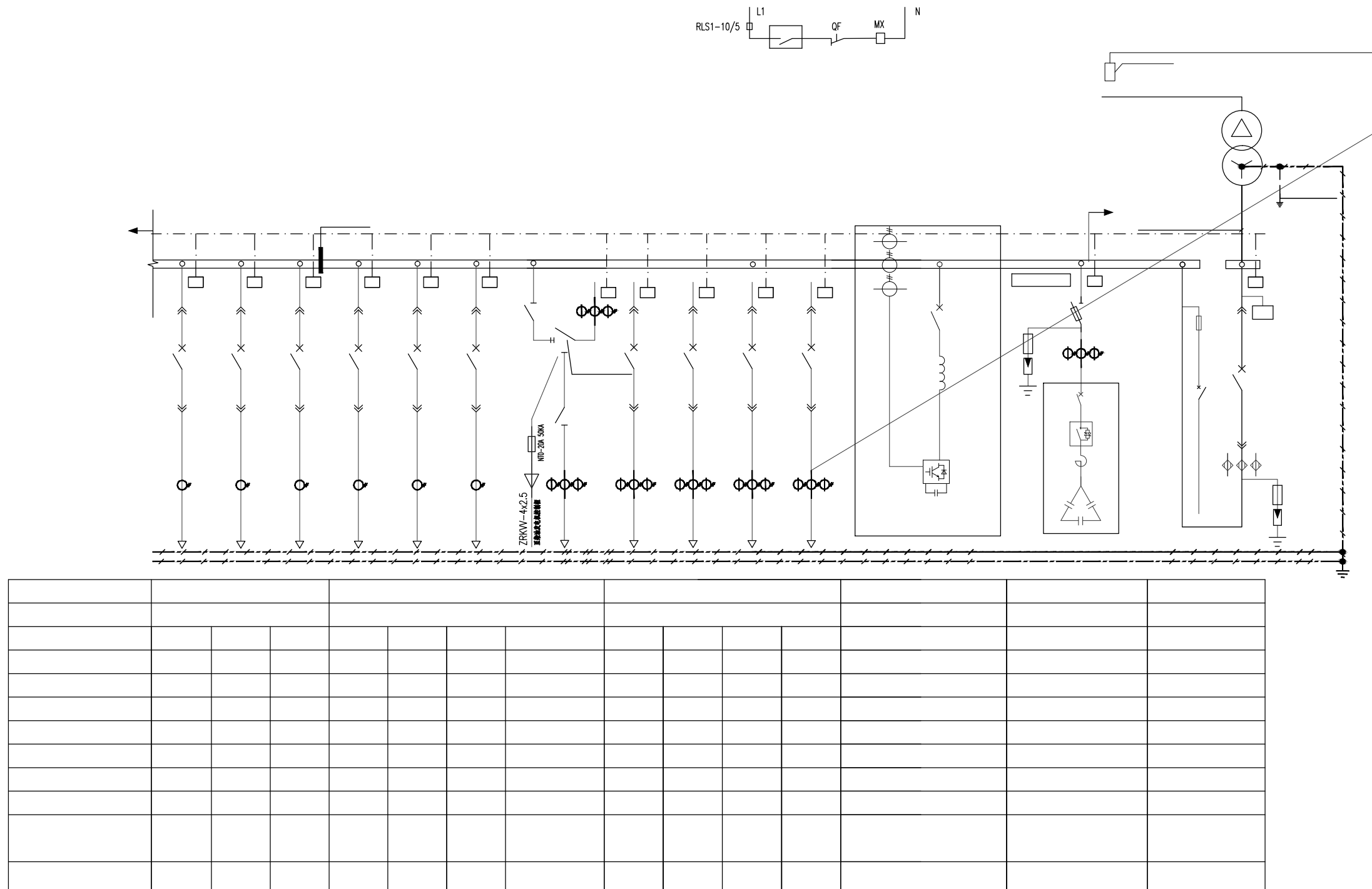
1T变压器低压配电系统图二
